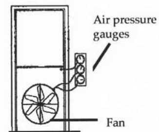
Blower Door
