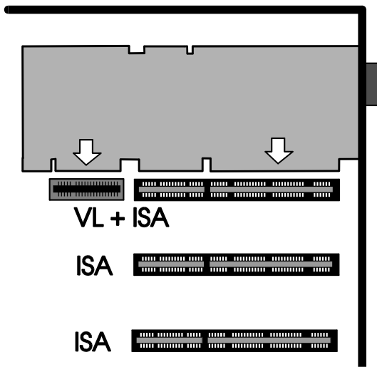
Installation in einem VESA Local Bus Erweiterungsslot
