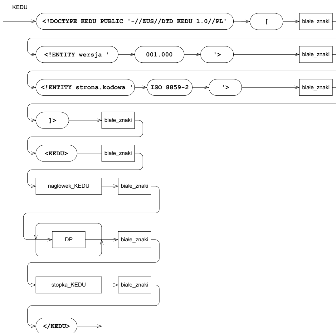
Diagram 1. Struktura KEDU
