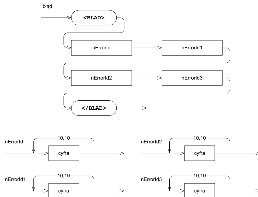
Diagram 8. Opis błędu
