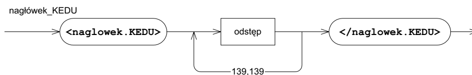
Diagram 2. Nagłówek KEDU
