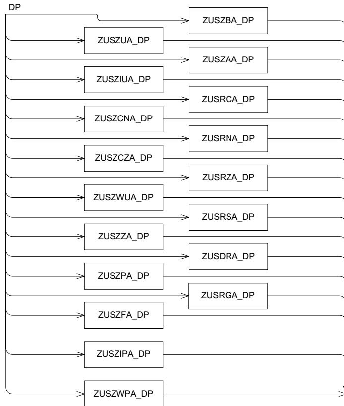
Diagram 4. Dokumenty płatnika
