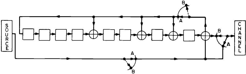
Fig. 7.10. Encoder #1 for a BCH code.
