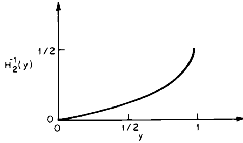
Fig. 10.9. The inverse function H_2^{-1}(y) .
