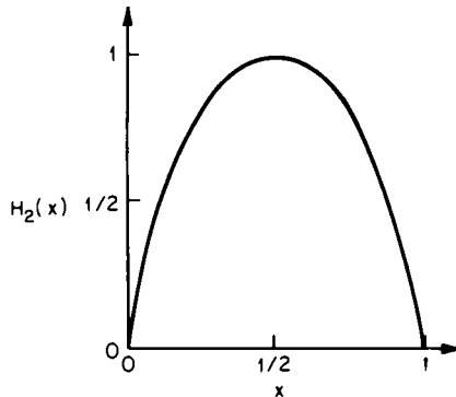
Fig. 10.8. The entropy function H_2(x) .
