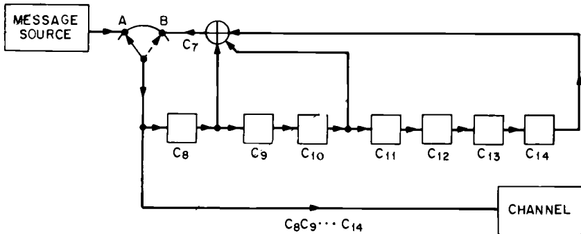
Fig. 7.11. Encoder #2 for a BCH code.
