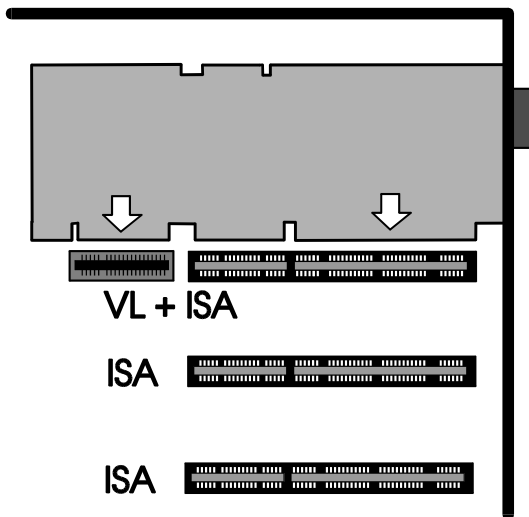
Installation in einem VESA Local Bus Erweiterungsst
