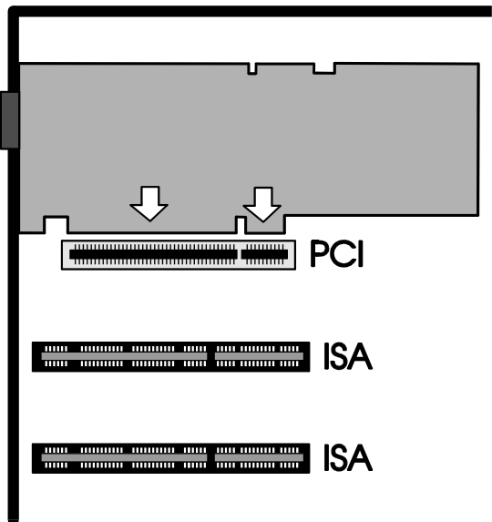
Installation in einem PCI Erweiterungsst
