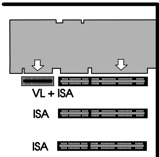
Instalación en una ranura de VL.
