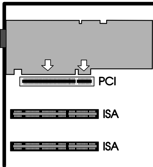
Instalación en una ranura de PCI.
