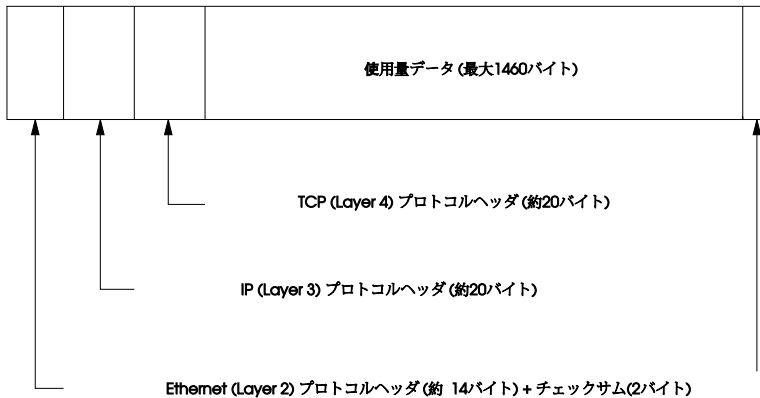
図 19.2 TCP/IPイーサネットパケット
