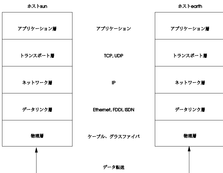
図 19.1 TCP/IPの簡易レイヤモデル
