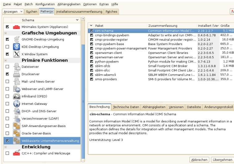
Abbildung 31.1 Paketauswahl für das Web-Based Enterprise Management-Muster
