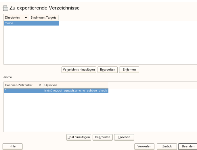
Abbildung 26.2 Konfigurieren eines NFS-Servers mit YaST
