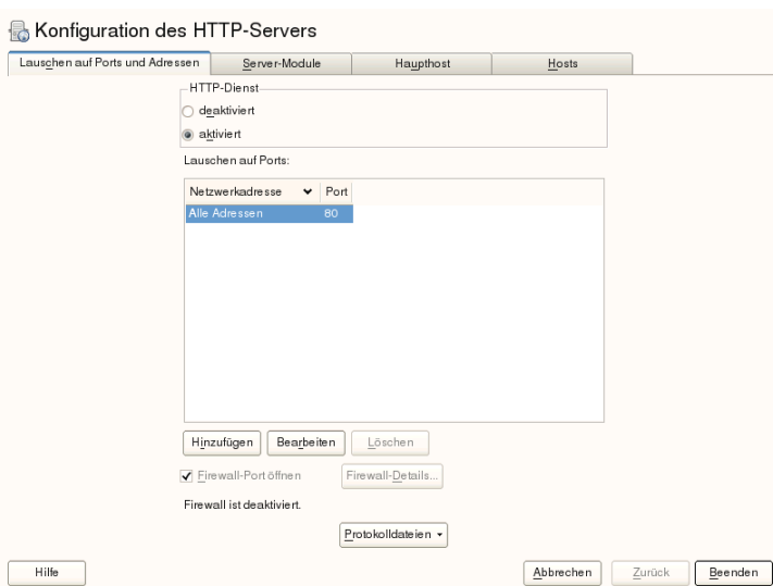
Abbildung 28.3 Konfiguration des HTTP-Servers: Überwachen von Ports und Adressen
