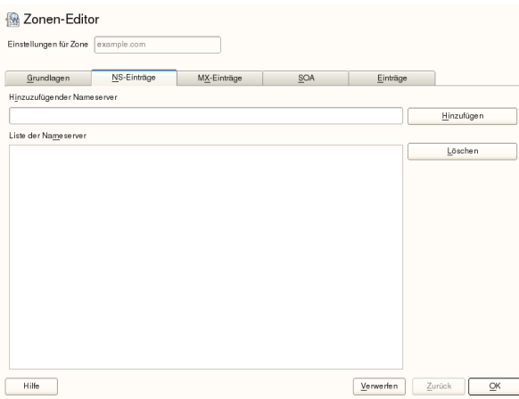
Abbildung 22.6 DNS-Server: Zonen-Editor (DNS-Einträge)
