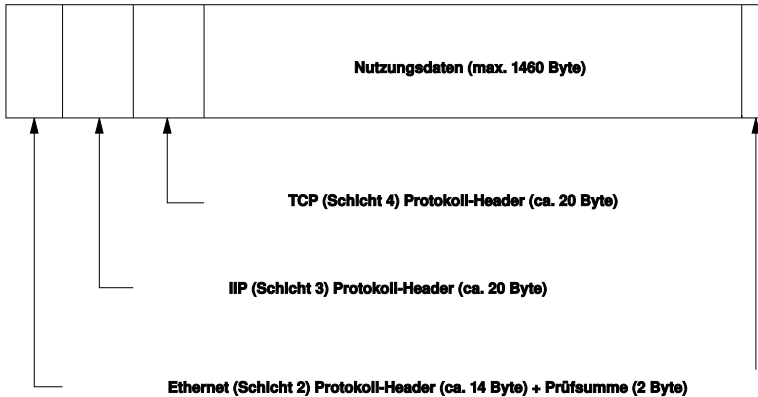
Abbildung 19.2 TCP/IP-Ethernet-Paket
