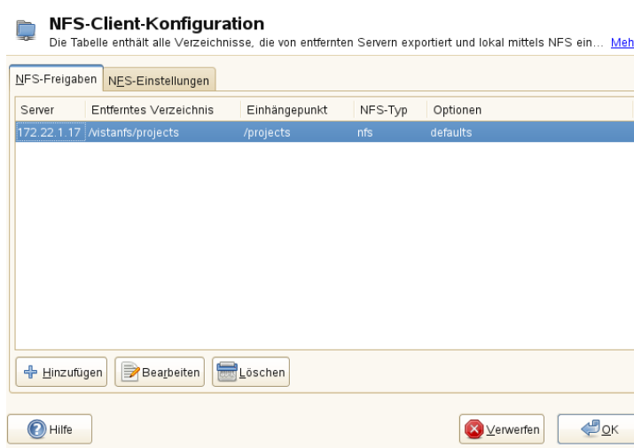
Abbildung 26.5 Konfiguration des NFS-Clients mit YaST
