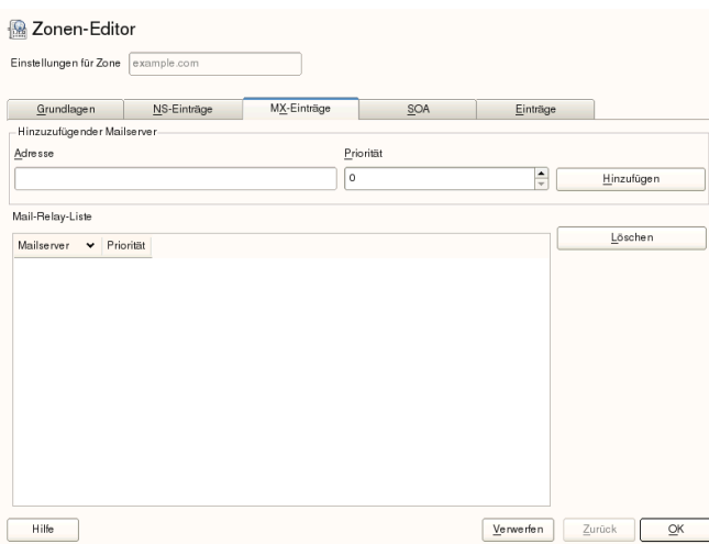
Abbildung 22.7 DNS-Server: Zonen-Editor (MX-Einträge)
