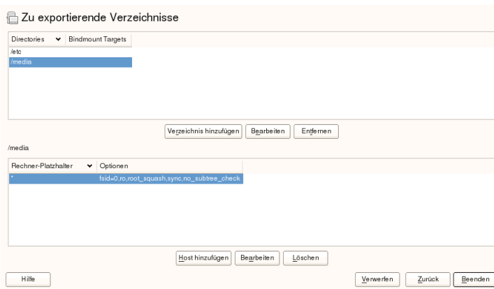
Abbildung 26.3 Exportieren von Verzeichnissen mit NFSv4
