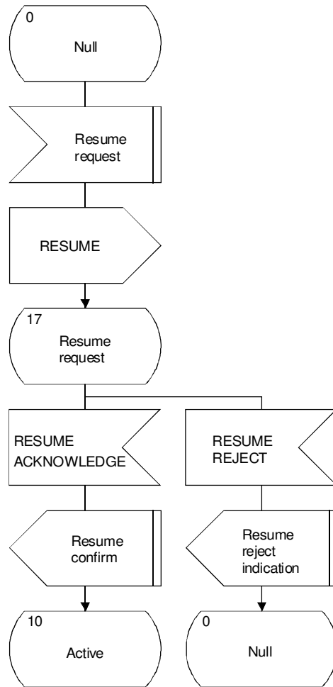
f) Resume procedure
